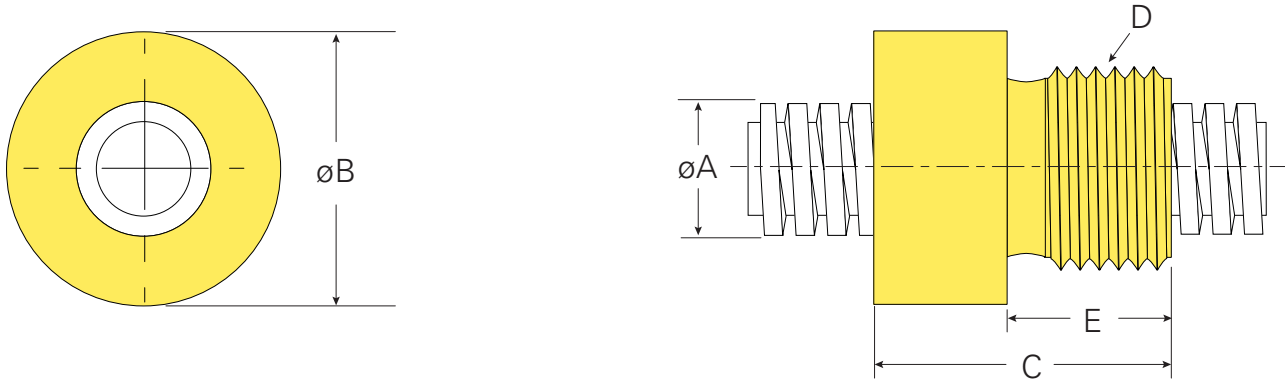
Nut
